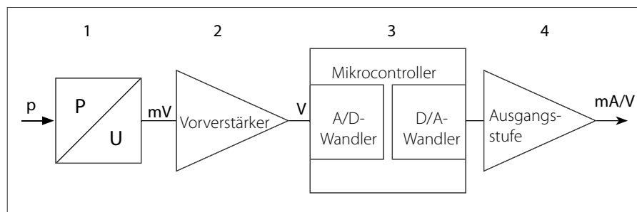
Blockschaltbild
